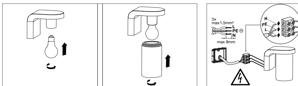
MONTAGE E27 LICHTBRON
