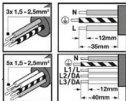
DP MAX bedradingschema
