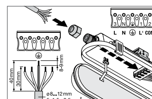
Aansluiting
