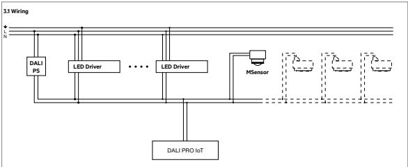
De sensor aansluiten op de DALI-bus
